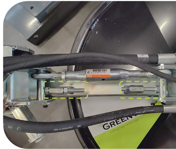
Position des vis de réglage de la fonction d'« inclinaison »
