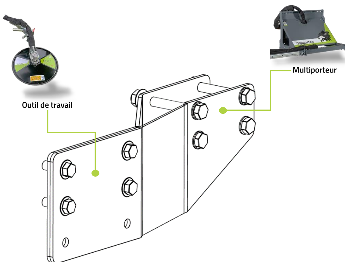
Fonction du support de base pour RI 62-82 ↔ FOX Multiporteur
