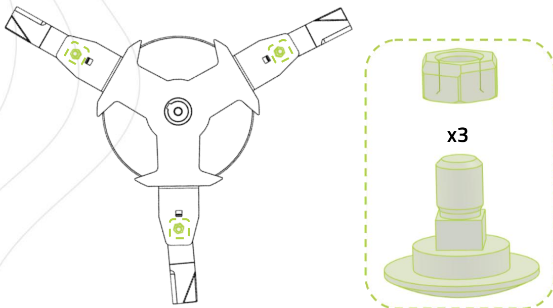
Dépose des boulons de lame (x3) sur le porte-lame
