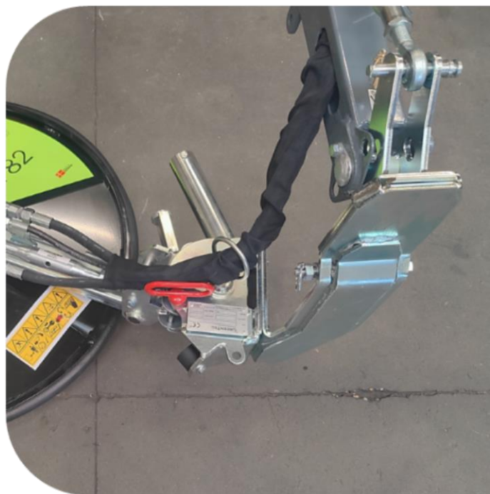
Adaptateur pour le montage : broyeur sous clôture RI ↔ PUMA 2303
