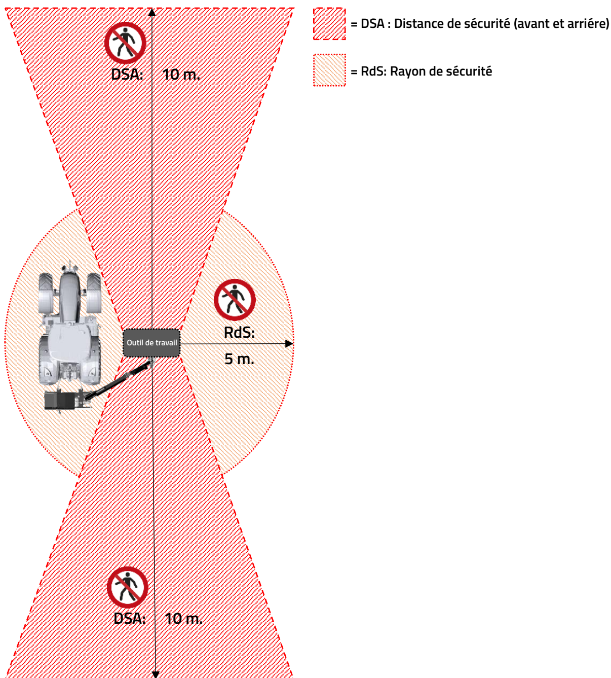
Figure 5 – Zones de sécurité (véhicule/outil de travail)
