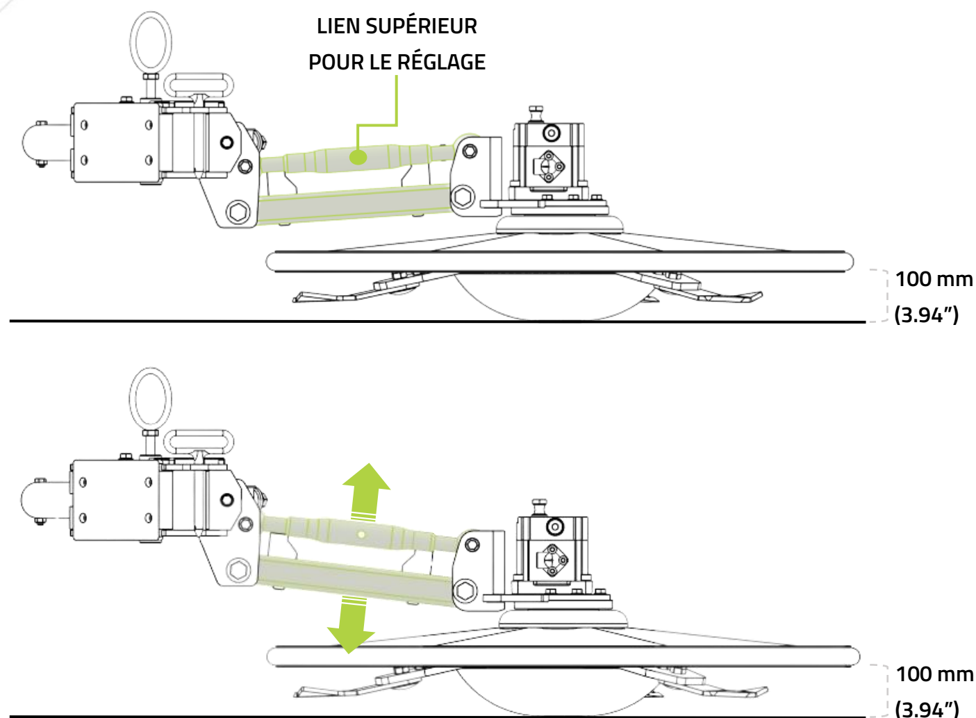
Fonction et réglage de la suspension : hauteur de travail
