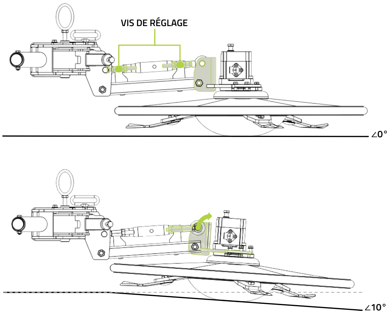
Fonction et réglage de la suspension : « fonction inclinaison »
