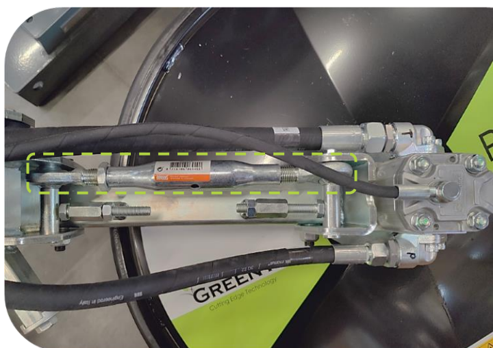
Position de l'articulation supérieure pour le réglage de la hauteur de travail de la suspension
