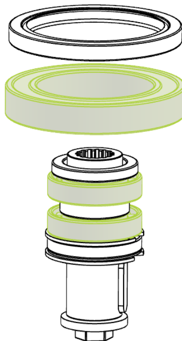
Roulements à billes sur l'arbre du rotor à pales
